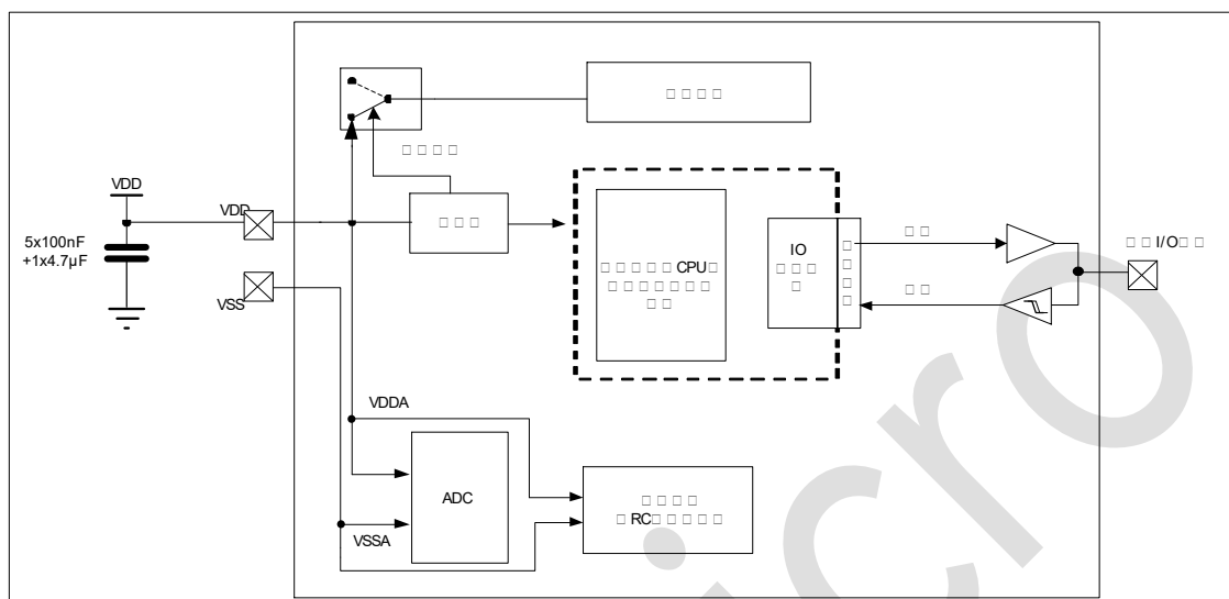
图 5-3：供电方案
