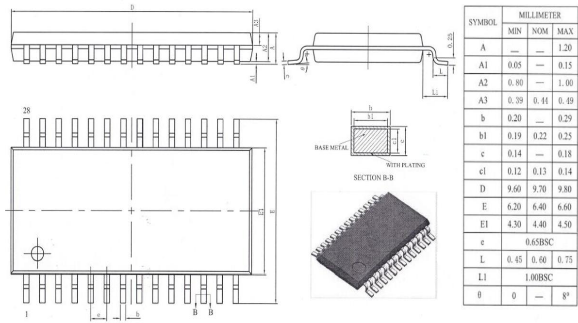
图 6-1: TSSOP28 封装尺寸图
